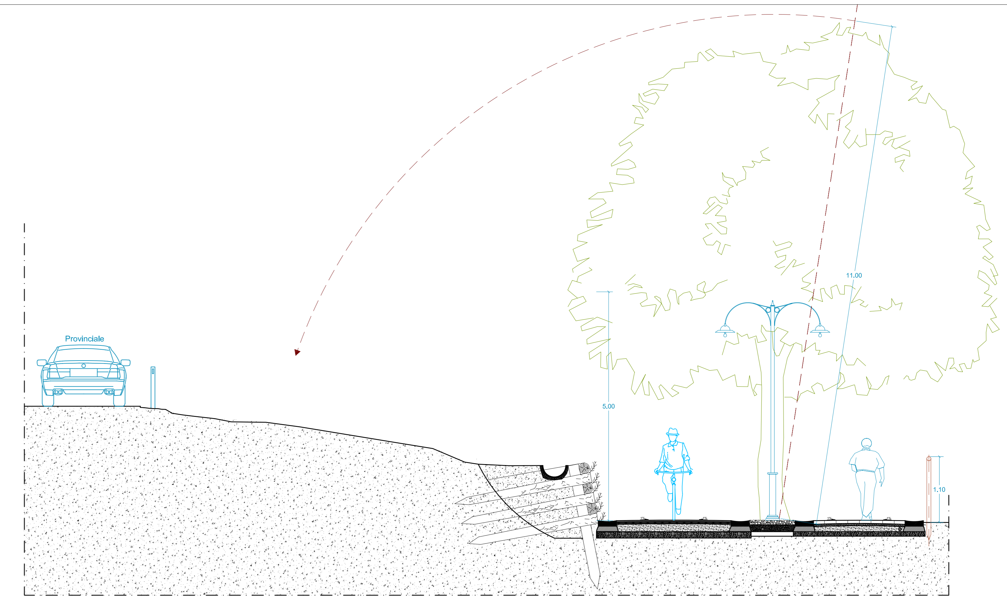
SEZ.2 Scala 1:50
