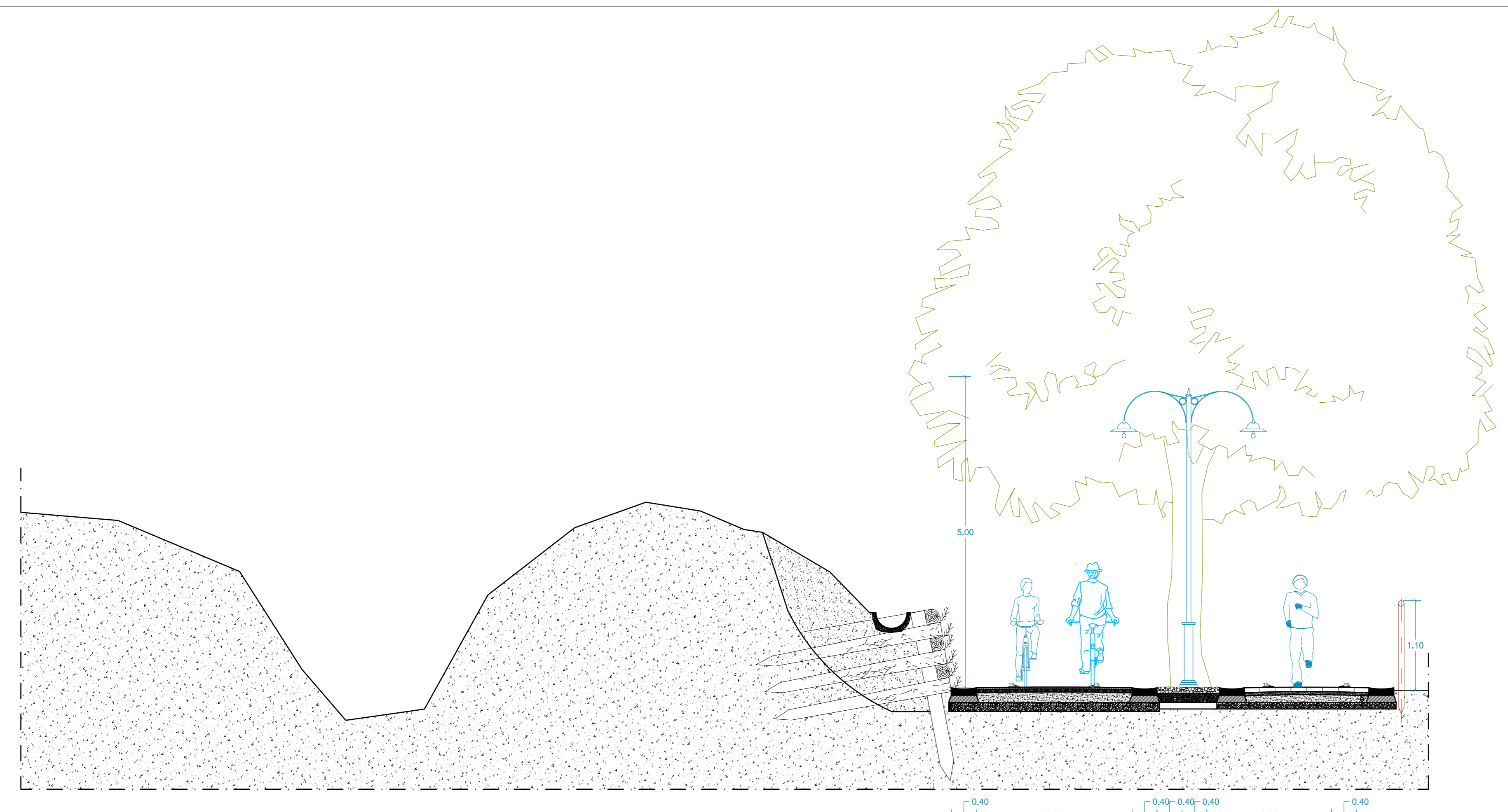
SEZ.3 Scala 1:50
