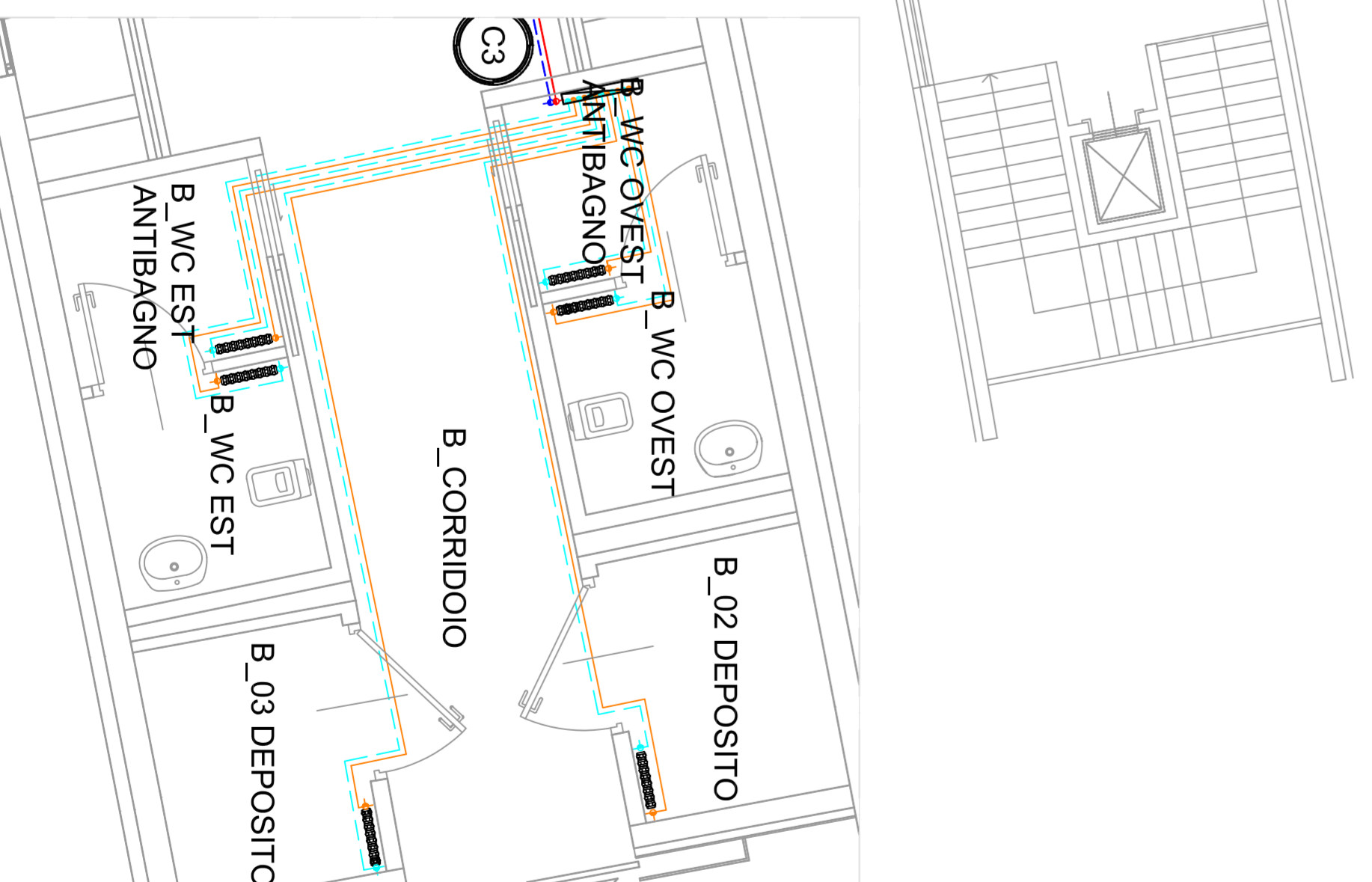
Particolare 2 - Servizi caffetteria - Scala 1:50
