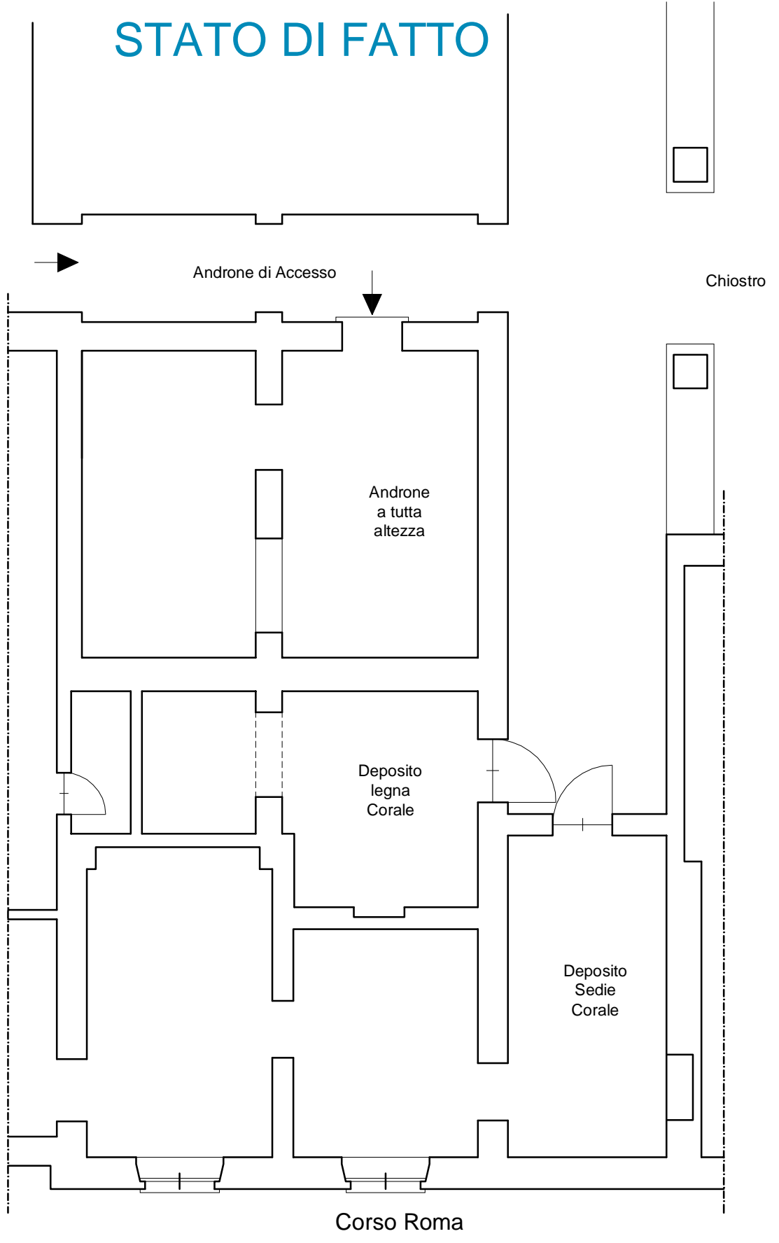
STATO DI FATTO PIANTA PORZIONE DI EX CASERMA CESARE BATTISTI Scala 1:100
